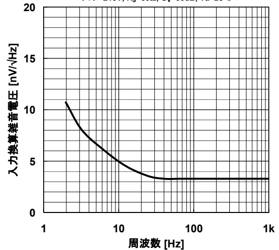
入力換算雑音電圧 対 周波数 特性例 V^+ / V^- = \pm 15V , R_s = 50\Omega , G_V = 60dB , T_a = 25^\circ C
