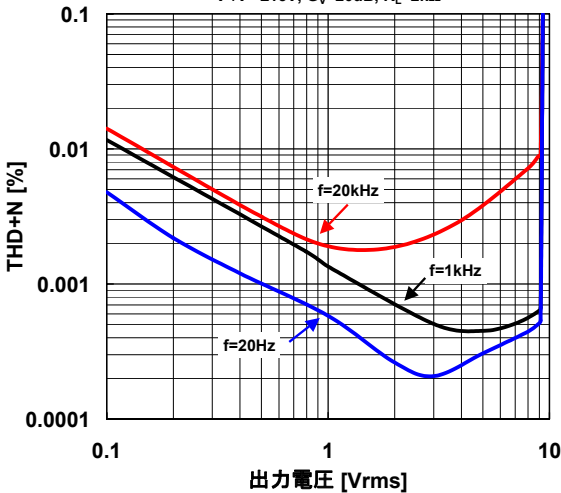
全高調波歪率 対 出力電圧 特性例 (周波数) V^+ / V^- = \pm 15V , G_V = 20dB , R_L = 2k\Omega
