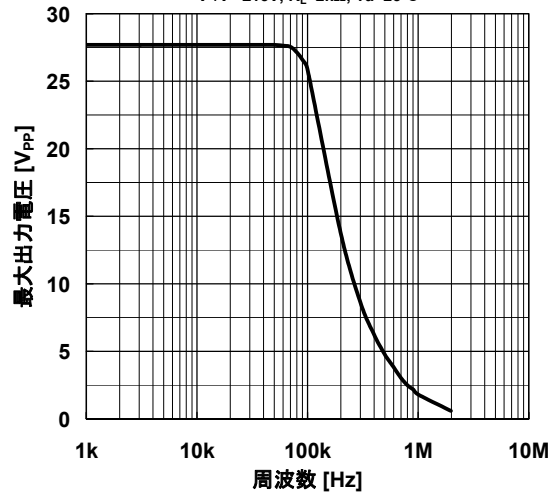
最大出力電圧 対 周波数 特性例 V^+ / V^- = \pm 15V , R_L = 2k\Omega , T_a = 25^\circ C
