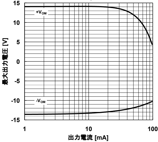
最大出力電圧 対 出力電流 特性例 V^+ / V^- = \pm 15V , T_a = 25^\circ C
