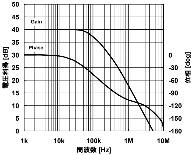
40dB 利得/位相 対 周波数 特性例 ( V^+ / V^- = \pm 15V , R_L = 2k\Omega , T_a = 25^\circ C )
