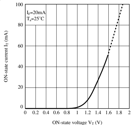
Fig.12 オン電流 オン電圧特性
