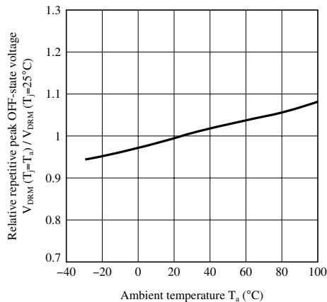
Fig.5 相对繰り返しピークオフ電圧 周囲温度特性
