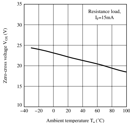
Fig.11 ゼロクロス電圧 周囲温度特性
