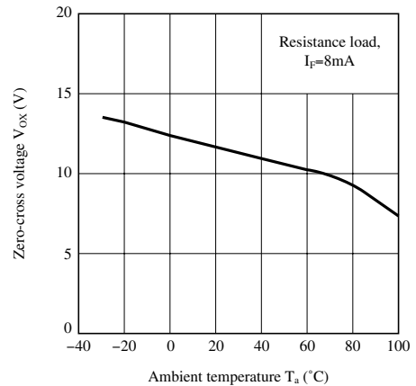
Fig.10 ゼロクロス電圧 周囲温度特性 (ランクC)
