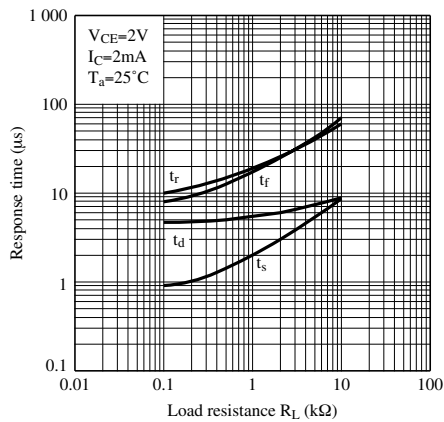
Fig.12 応答時間—負荷抵抗特性
