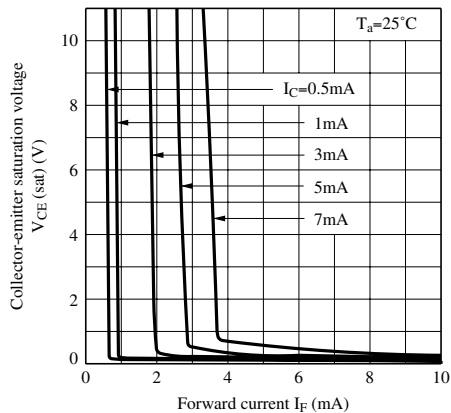
Fig.14 コレクタ・エミッタ間飽和電圧— 順電流特性
