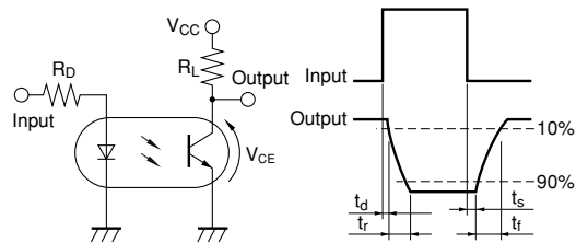
Fig.13 応答時間の測定回路
