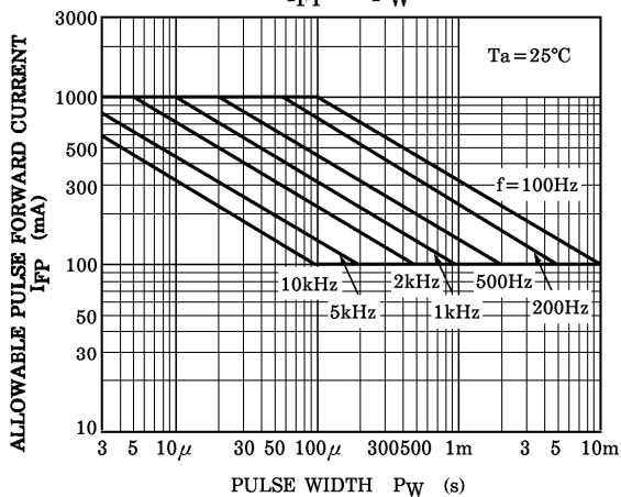
I_{FP} - P_W
