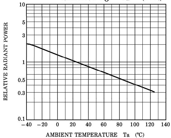
RELATIVE P_O - T_a (TYP.)
